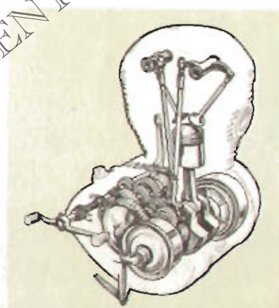
Transmission primaire par engrenages hélicoïdaux parfaitement silencieux. Boîte à 4 vitesses avec point mort verrouillé.
