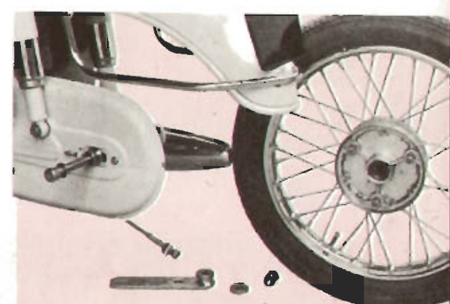
Roue arrière facilement démontable grâce à son moyeu à broche. Freins à tambour central, rayonnage renforcé, amortisseur de transmission.
