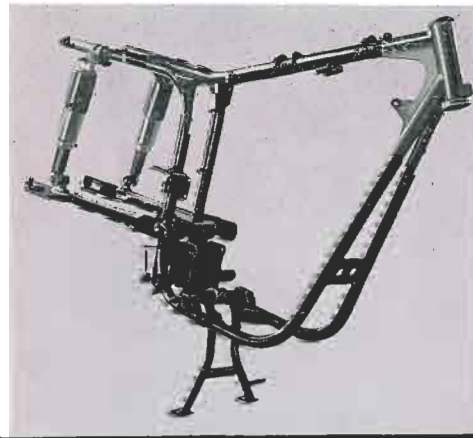
Cadre en double berceau d'une rigidité absolue. Fourche avant télescopique, suspension arrière oscillante avec amortisseurs.
